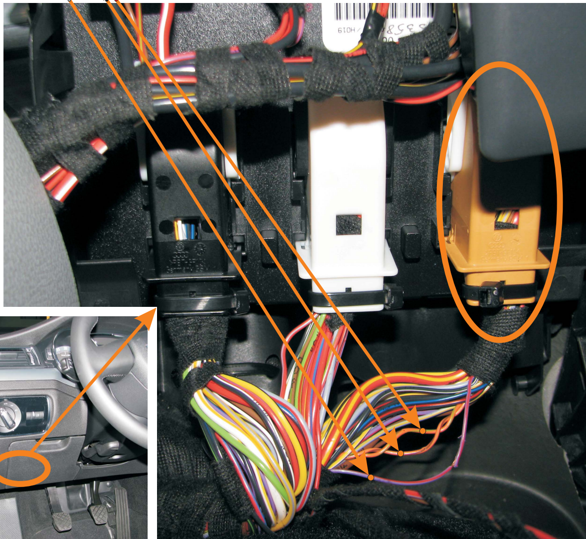
KOLEJNOŚĆ PODŁĄCZANIA PRZEWODÓW: MASA, +12V, CANL, CANH ...
