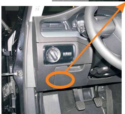
KOLEJNOŚĆ PODŁĄCZANIA PRZEWODÓW: MASA, +12V, CANL, CANH ...
