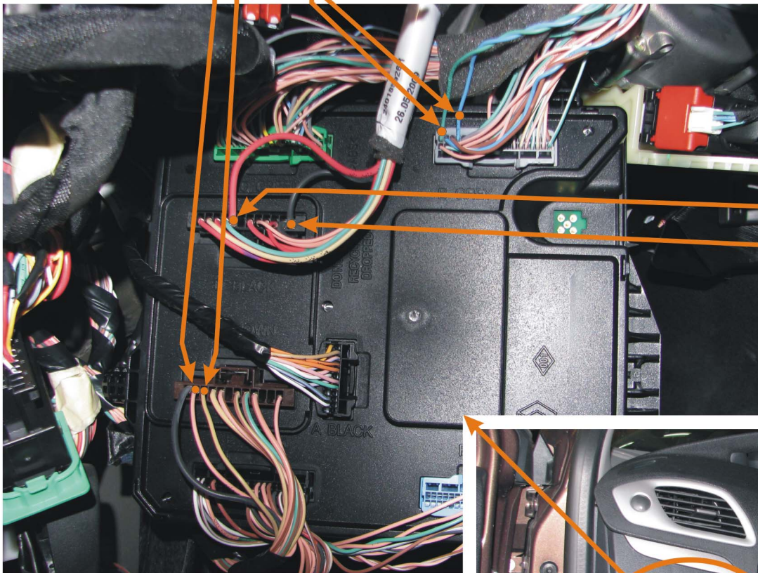
+12V czerwony pin8 czarne złącze "D" 12PIN MASA czarny pin1 czarne złącze "D" 12PIN
