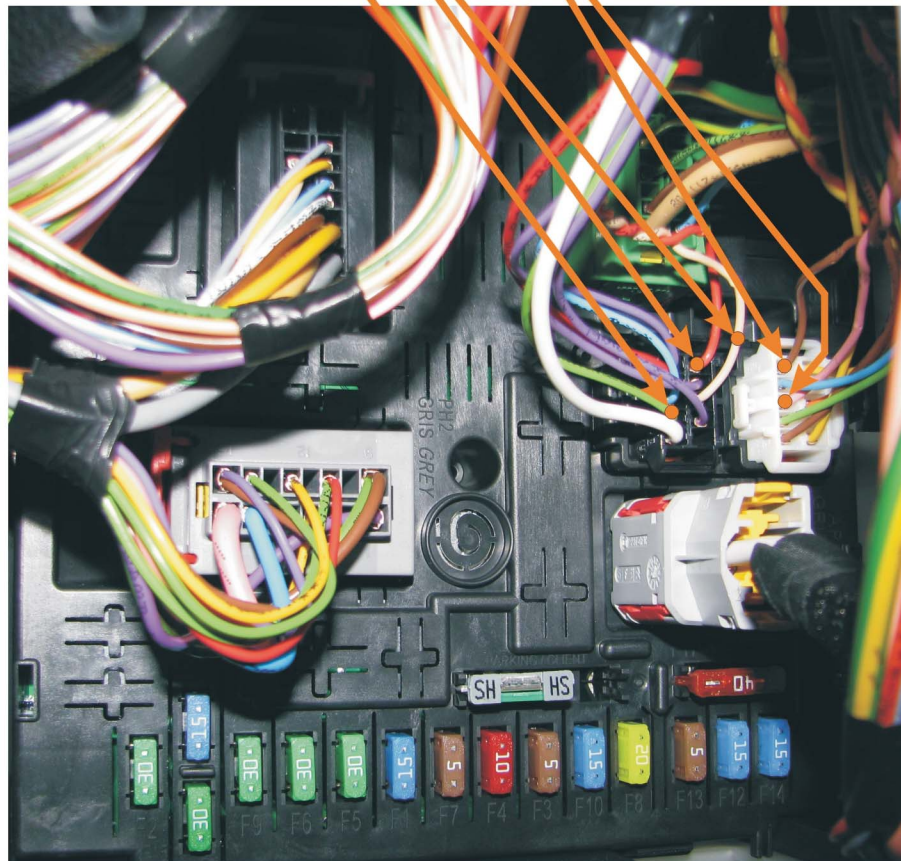
KOLEJNOŚĆ PODŁĄCZANIA PRZEWODÓW: MASA, +12V, CANL, CANH ...
