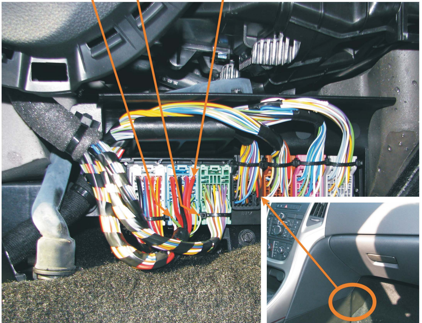
KOLEJNOŚĆ PODŁĄCZANIA PRZEWODÓW: MASA, +12V, CAN ...
