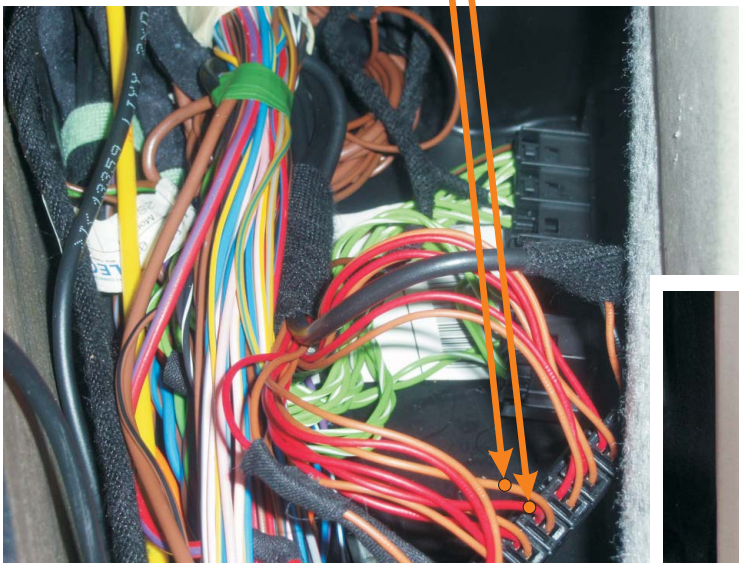
LISTWA ŁĄCZEŃ MAGISTRALI CAN (w progu kierowcy)
