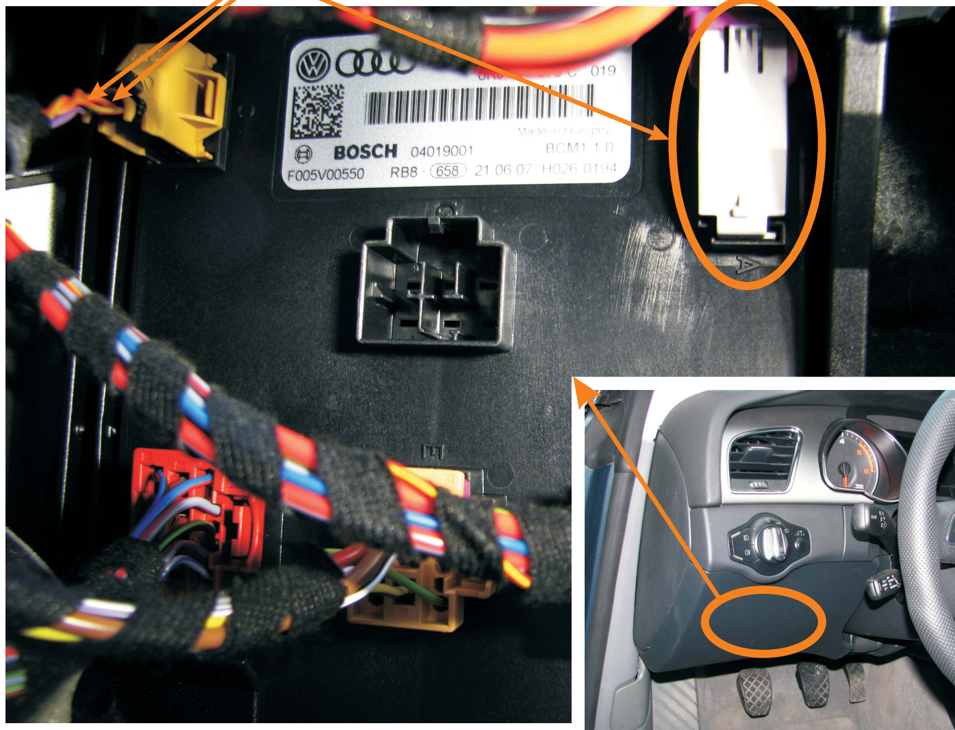
KOLEJNOŚĆ PODŁĄCZANIA PRZEWODÓW: MASA, +12V, CANL, CANH ...
