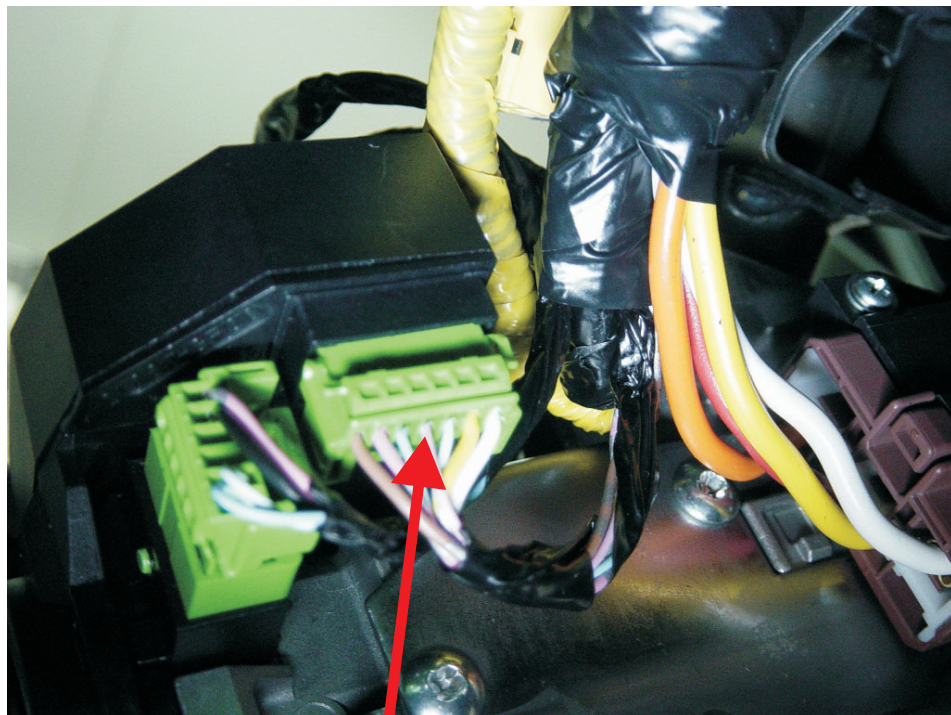
Różowy ( PIN4) - CAN H
