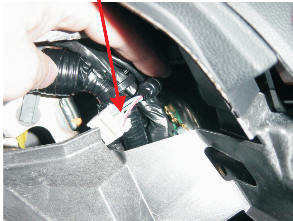
Zielony - włączanie świateł awaryjnych (+)
