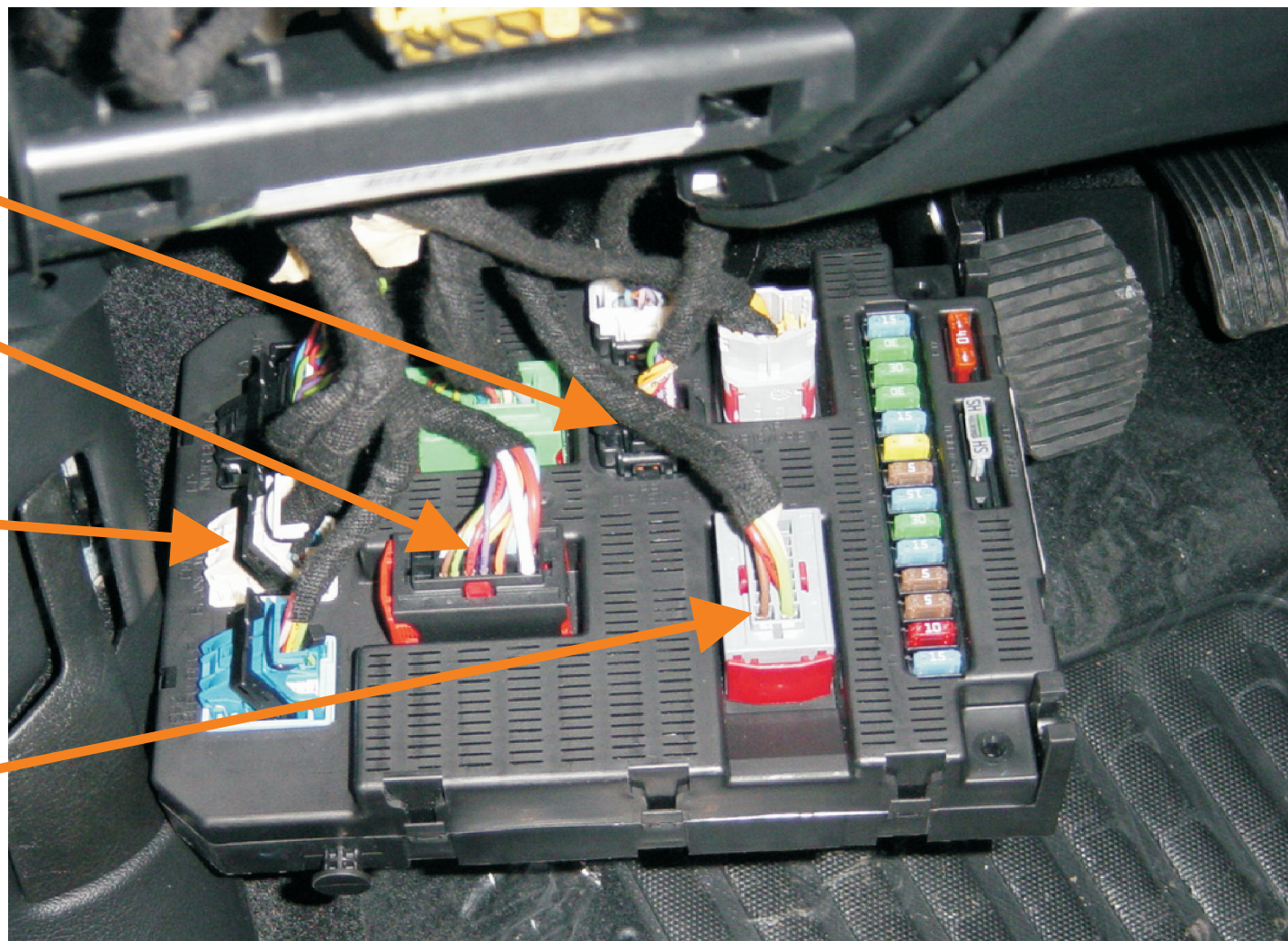
Moduł sterujący z lewej strony kolumny kierownicy
